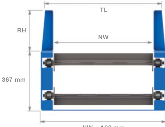
Coupe B-B
